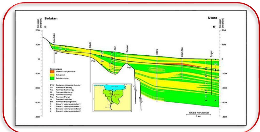
Gambar I-3 Potongan Melintang Selatan-Utara di Provinsi DKI Jakarta
