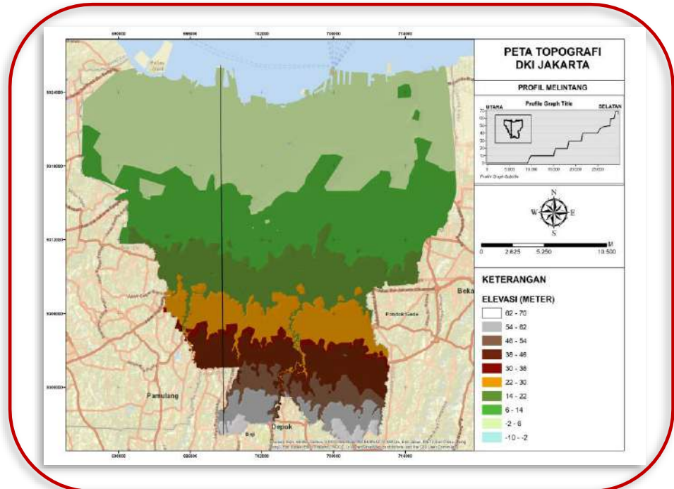
Gambar I-4 Topografi di Provinsi DKI Jakarta
