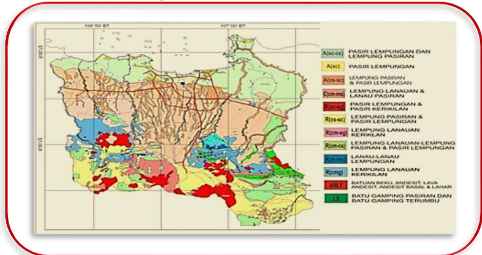
Gambar I-2 Morfologi Tanah di Provinsi DKI Jakarta
